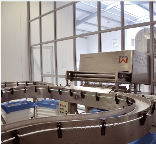
Cooling Machine 冷却机
