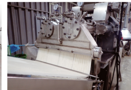
Vermicelli Extruder 挤丝机
