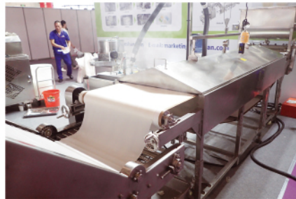
Steaming Machine 蒸粉机
