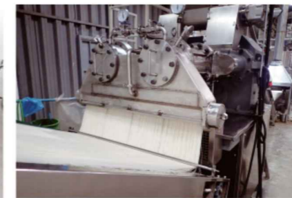
Vermicelli Extruder 挤丝机
